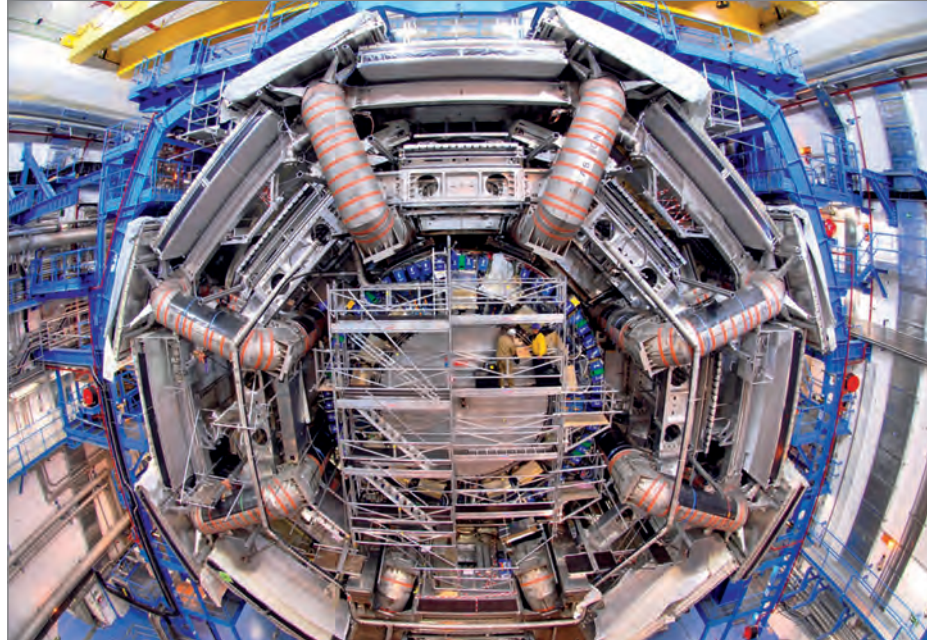
Detector ATLAS durante la fase de ensamblado en la caverna situada a 100 metros de profundidad bajo tierra.
