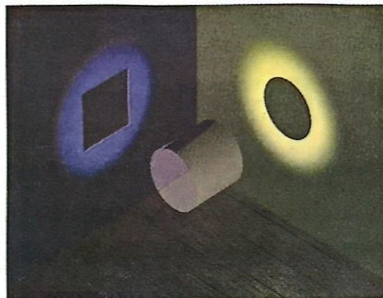
Imagen ilustrativa de la dualidad onda-partícula, en la que se aprecia cómo un mismo fenómeno puede ser percibido de dos modos distintos. Wikipedia
